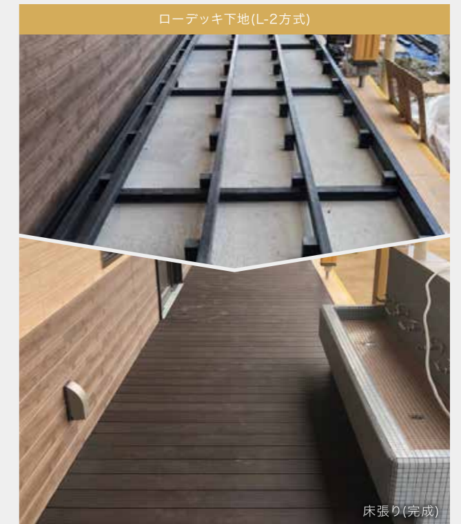
床張り(完成)
