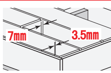
床板幅方向の隙間
