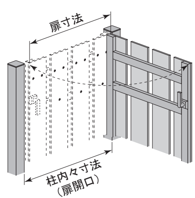
□吊元が右、後開きの場合
