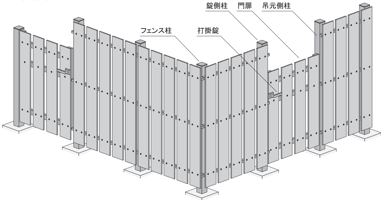
□吊元が左、前開きの場合
