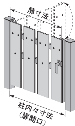
□吊元が左、前開きの場合
