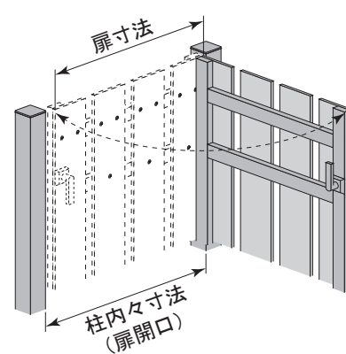
□吊元が右、後開きの場合
