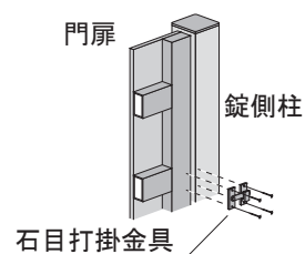
□石目打掛金具の場合
