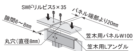
□笠木用パネルW100の場合
