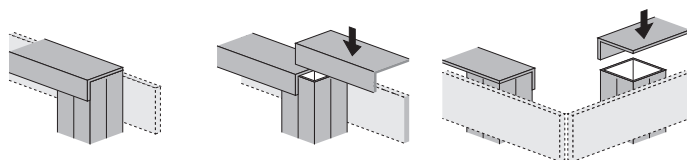
アルミ柱75×75
